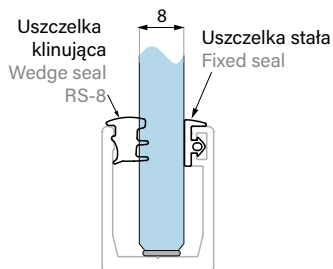
8mm szkło / glass RS-8+UNISEAL
