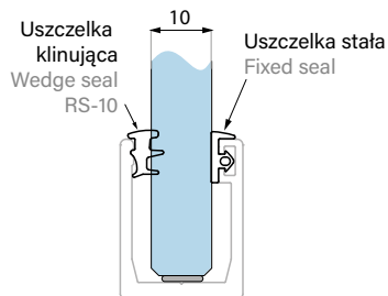
10mm szkło / glass RS-10+UNISEAL
