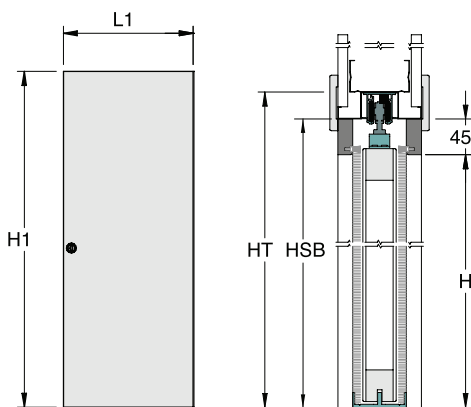
Runkoelementin rakenne ja mitat
